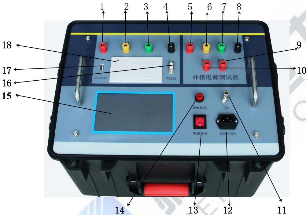
图 2 面板示意图
